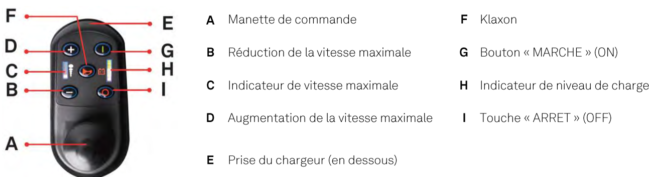
Illustration 2 : vue d'ensemble du boîtier de commande
