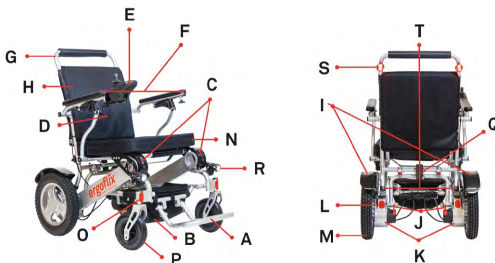
Illustration 1: vue d'ensemble du fauteuil roulant ergoflix L
