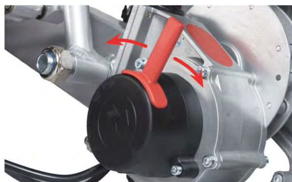
Illustration 11 : activation ou désactivation des freins électromagnétiques
